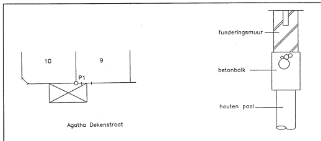
Type funderingsdetail
