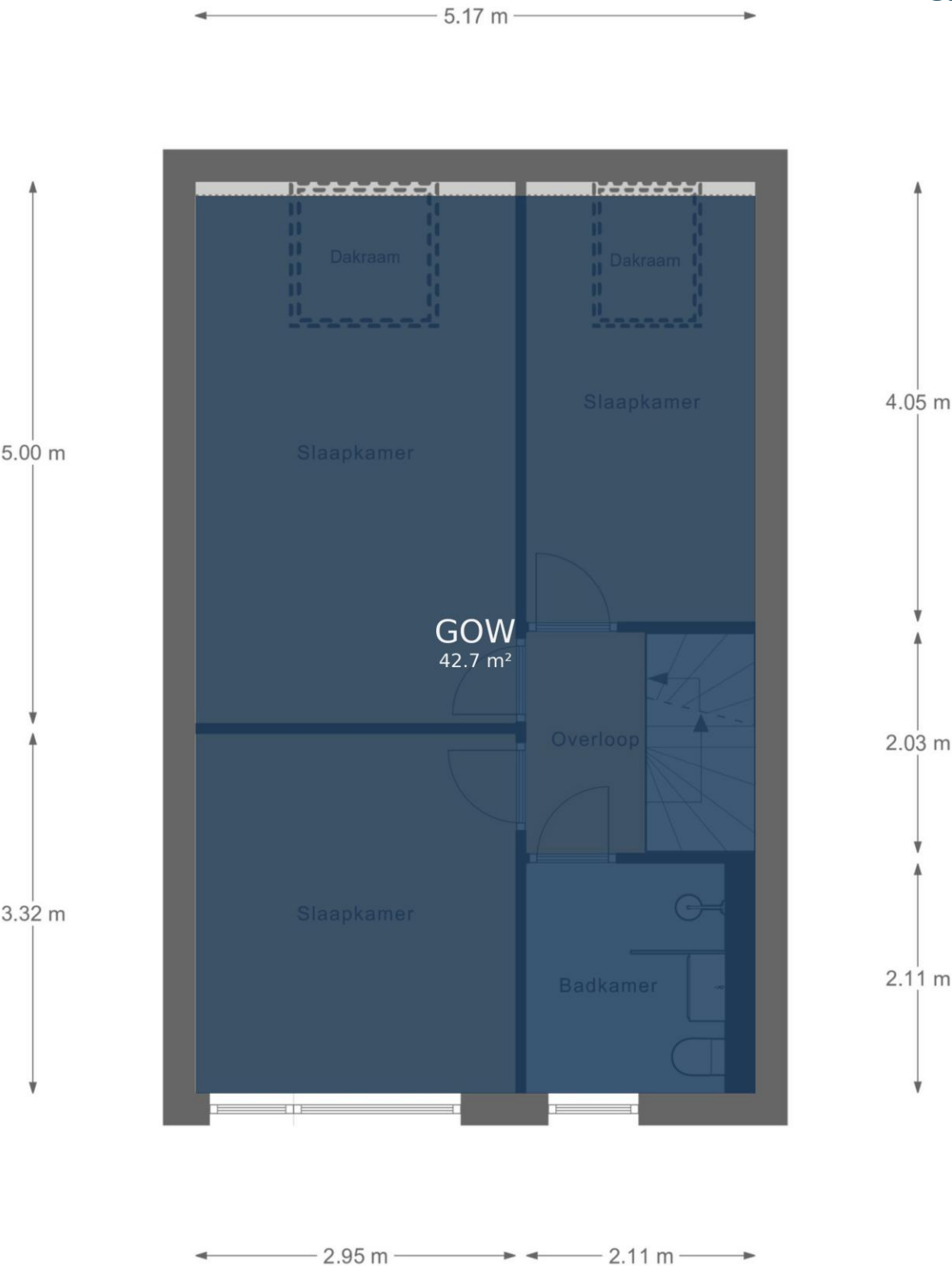
1e Verdieping
