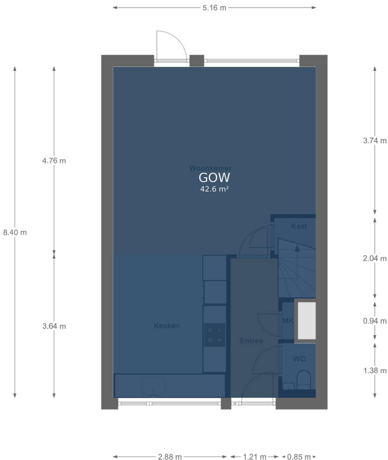
Begane Grond
