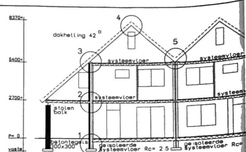
DOORSNEDE A-A
