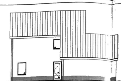
ZIJGEVEL VAN DER HEIJDEN
