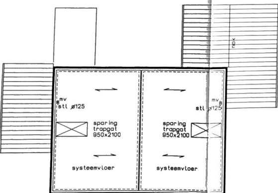
ZOLDERVLOER
