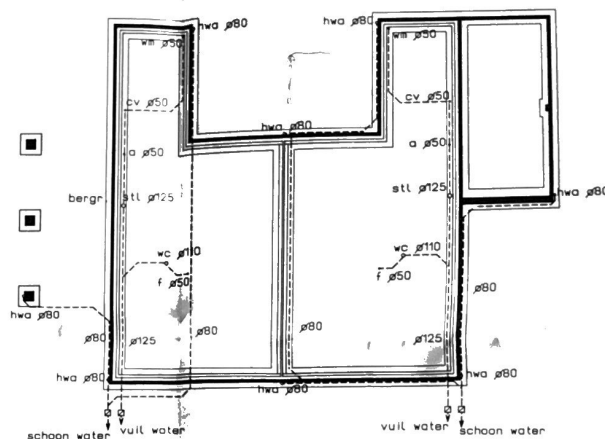
riolering aansluiten op bestaand riool FUNDERING/RIOIERING
