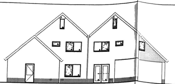
ACHTERGEVEL
