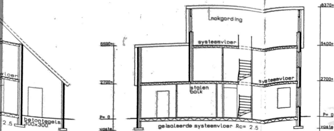
DOORSNEDE B-B
