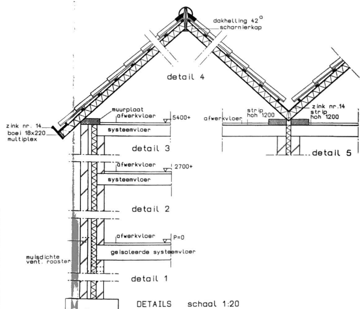
DETAILS schaal 1:20
