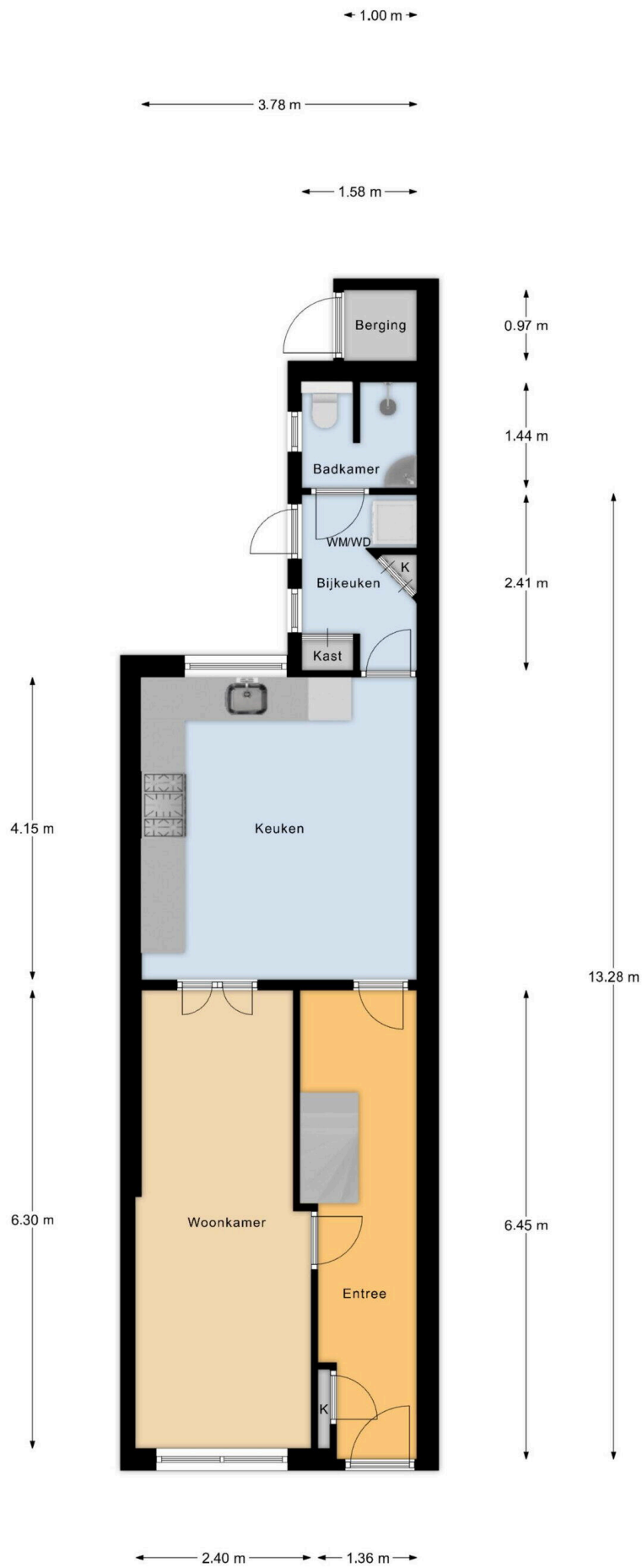
Begane Grond
