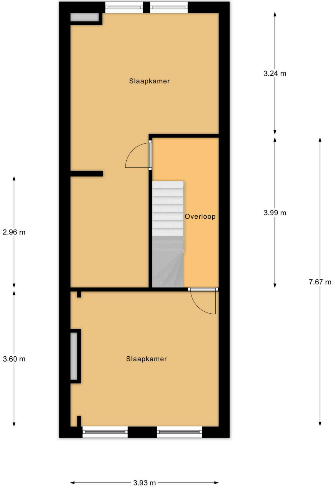
1e Verdieping
