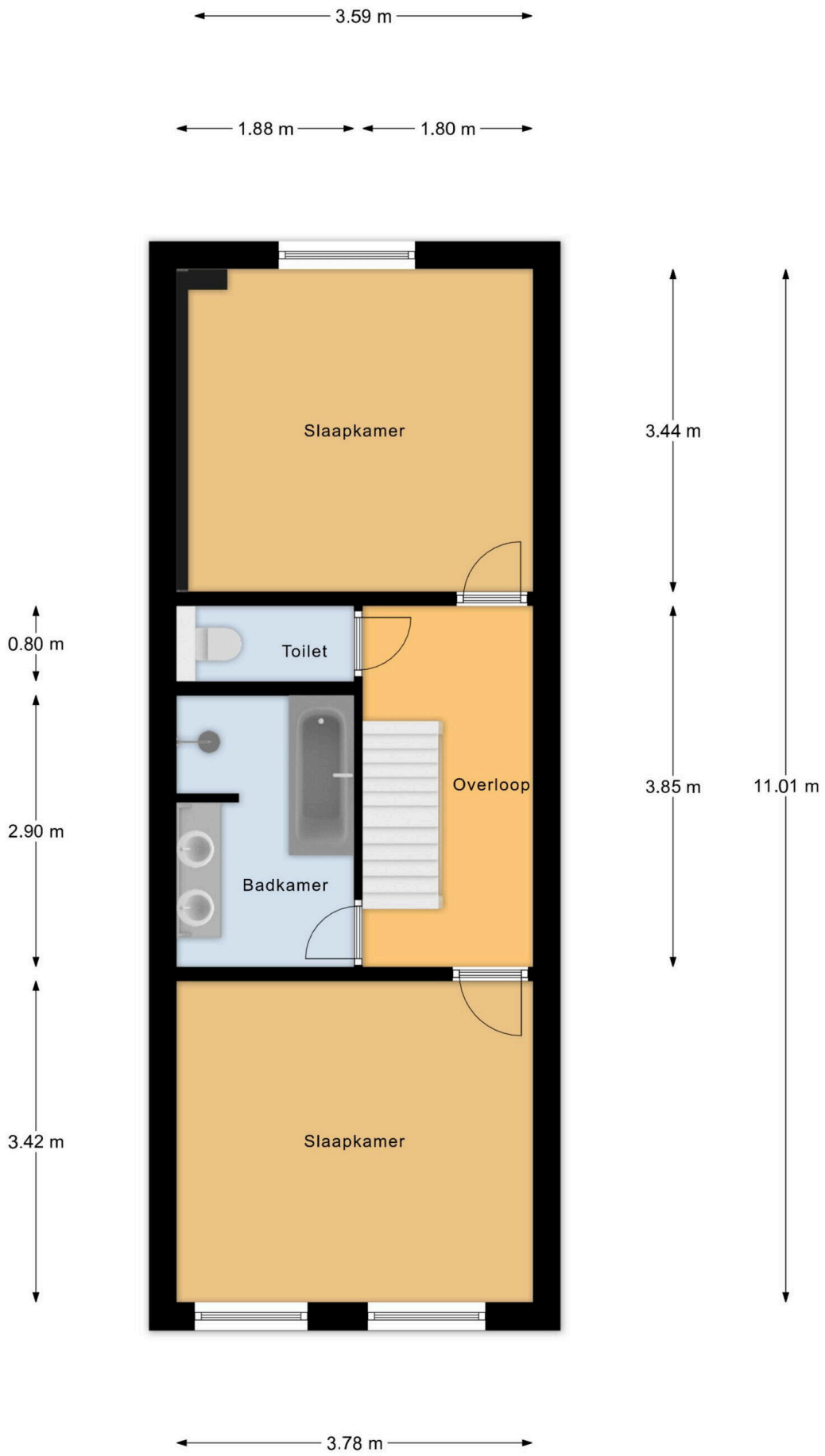
2e Verdieping
