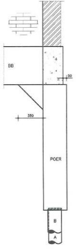
DOORSNED E A-A
