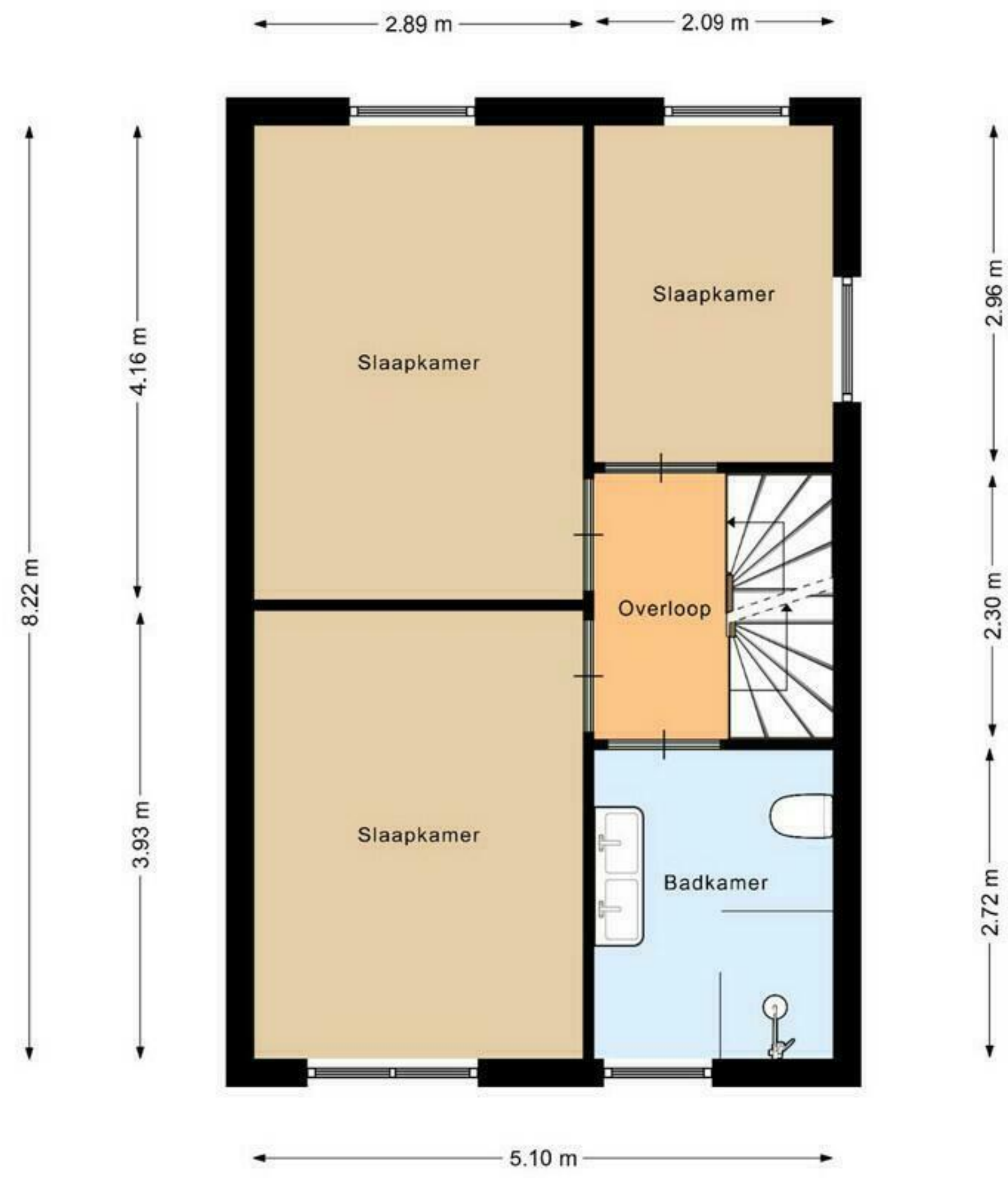
1e Verdieping
