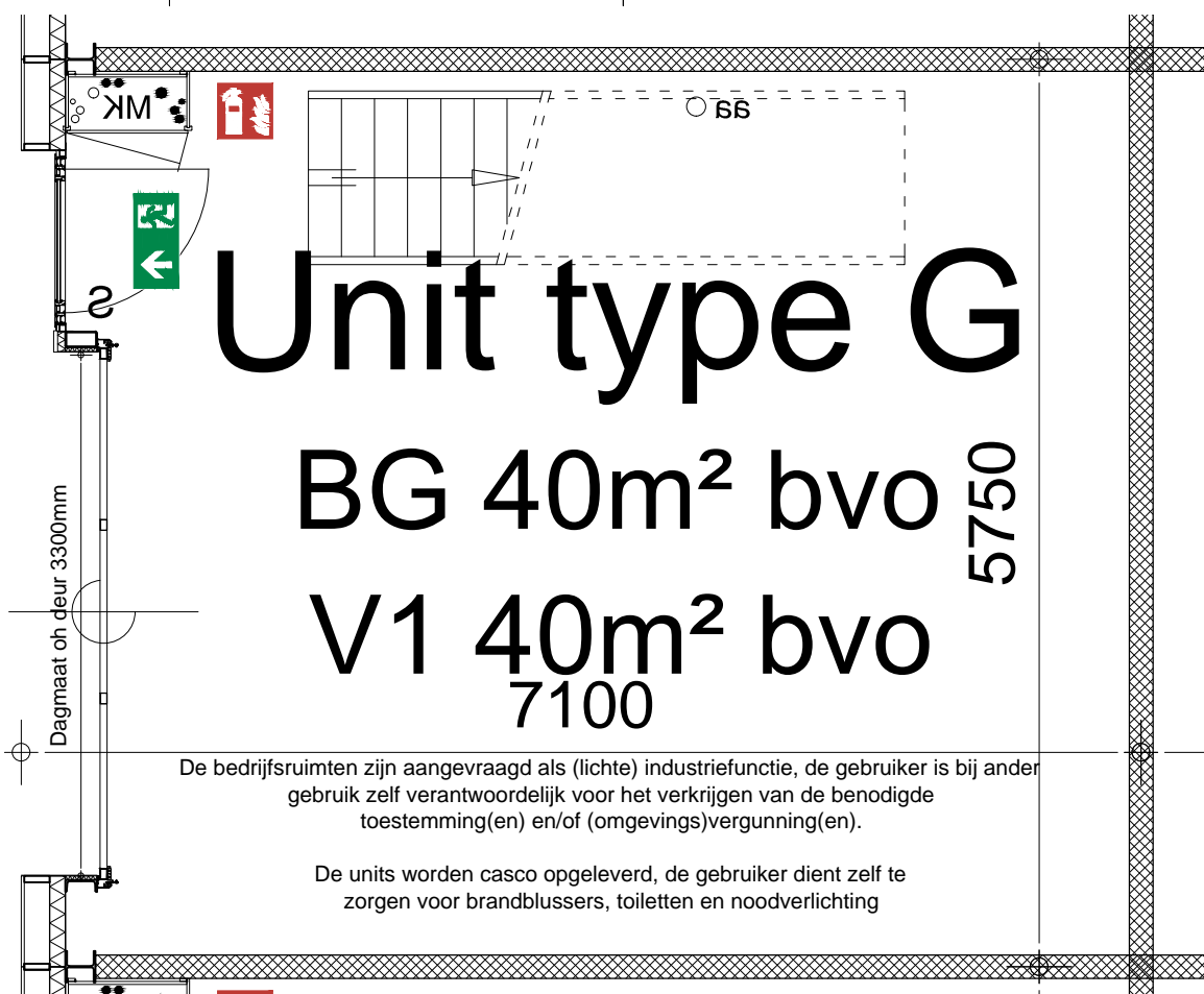
begane grond bedrijfsunit type G schaal 1:50
