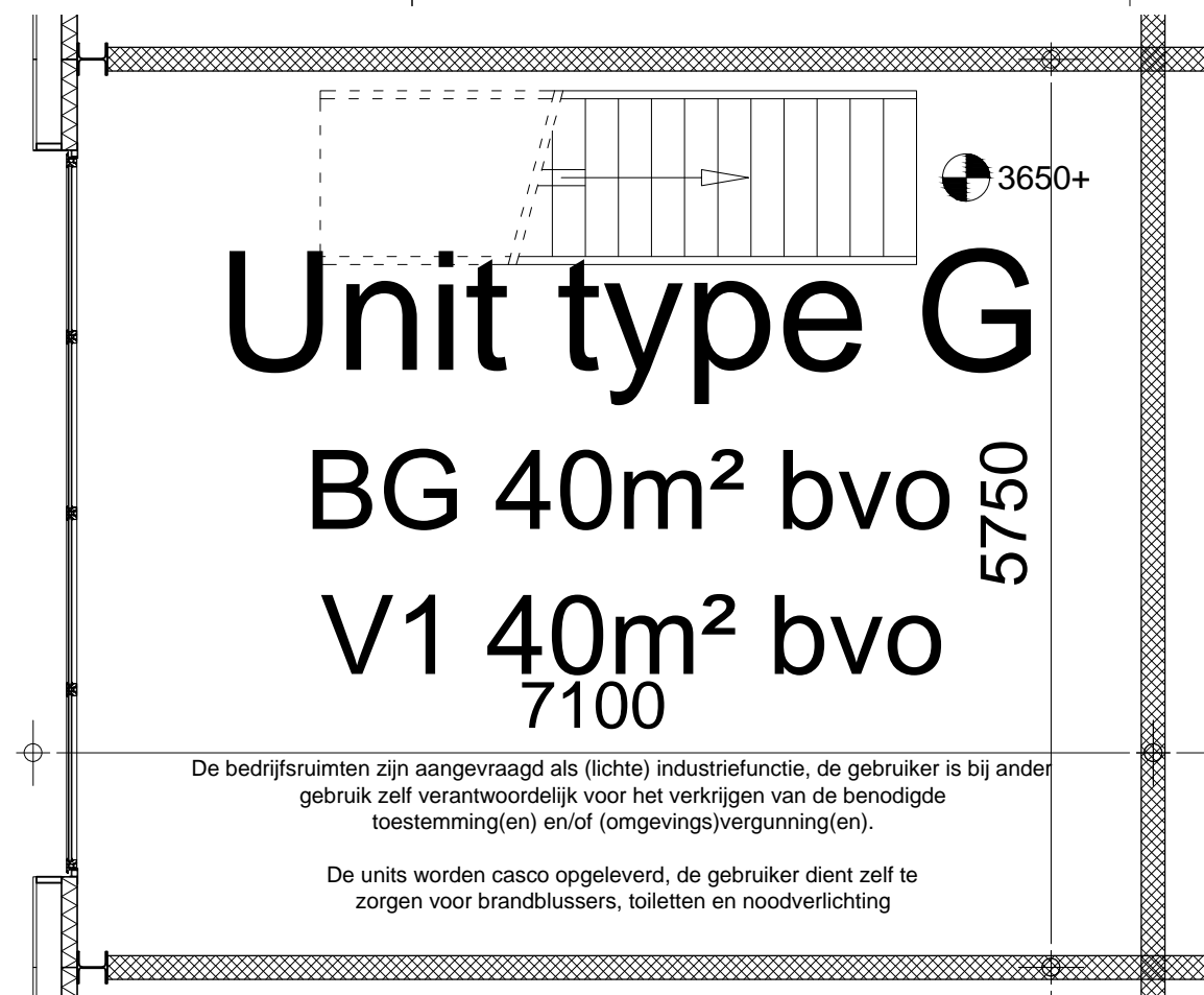
verdieping bedrijfsunit (3650+) type G schaal 1:50
