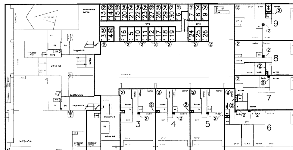
BEGANE GROND ~ 1 : 200
