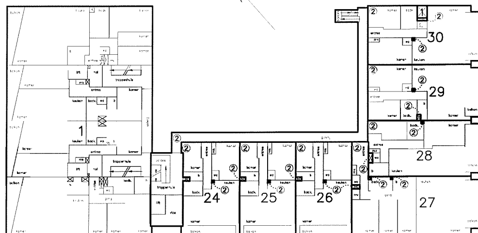
3e VERDIEPING ~ 1 : 200
