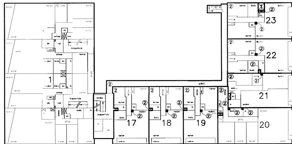
2e VERDIEPING ~ 1 : 200
