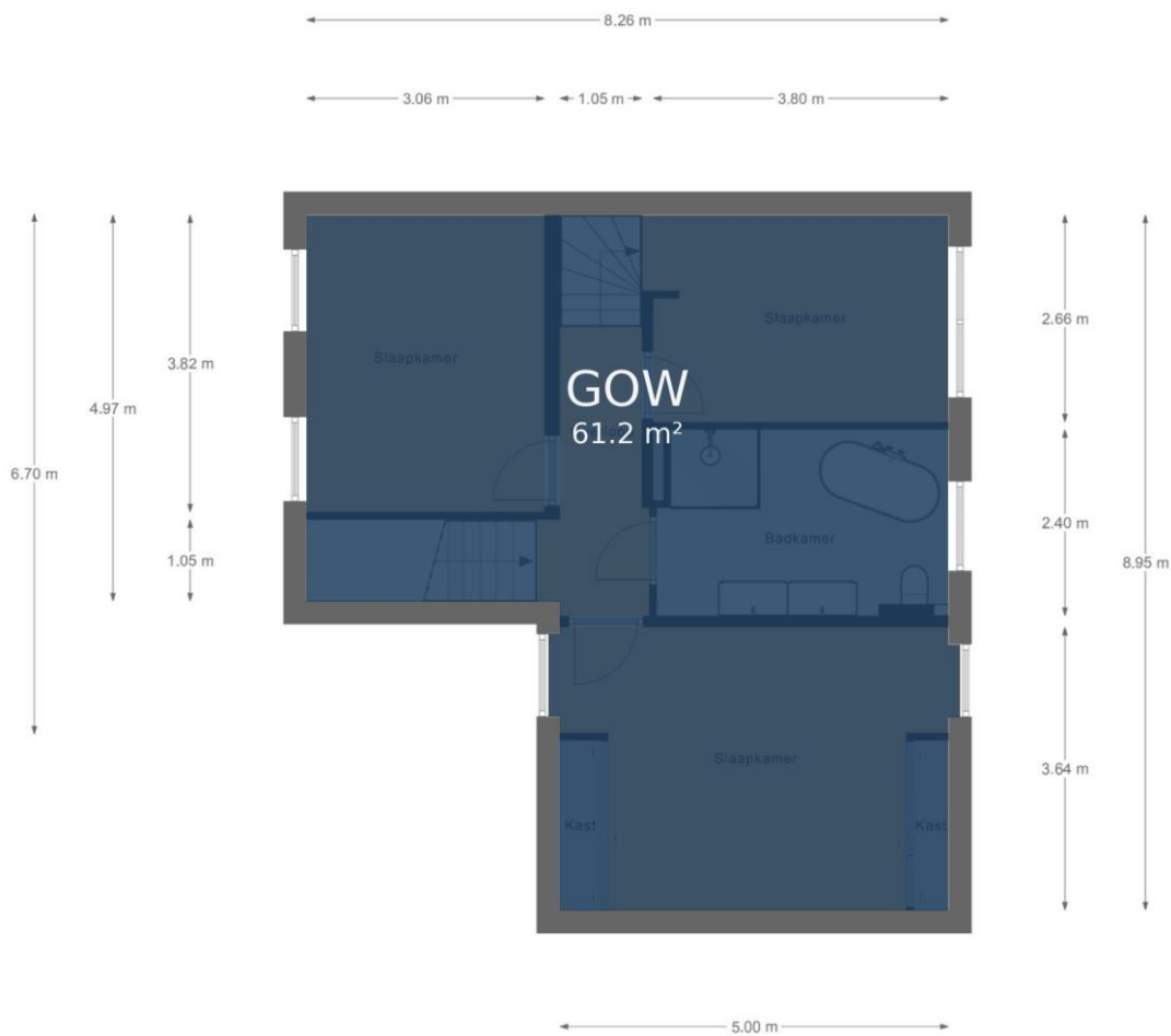
1e Verdieping
