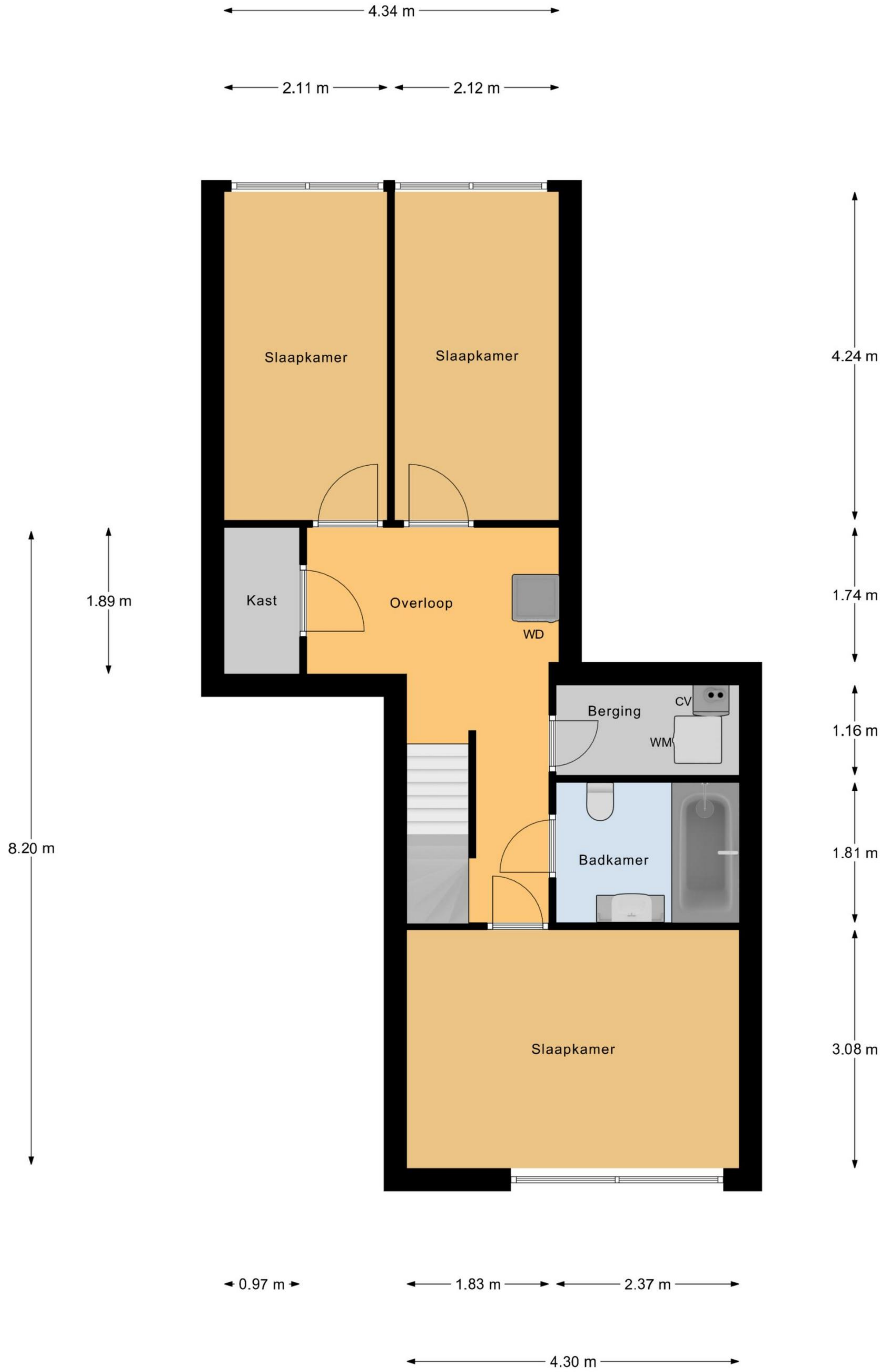
1e Verdieping
