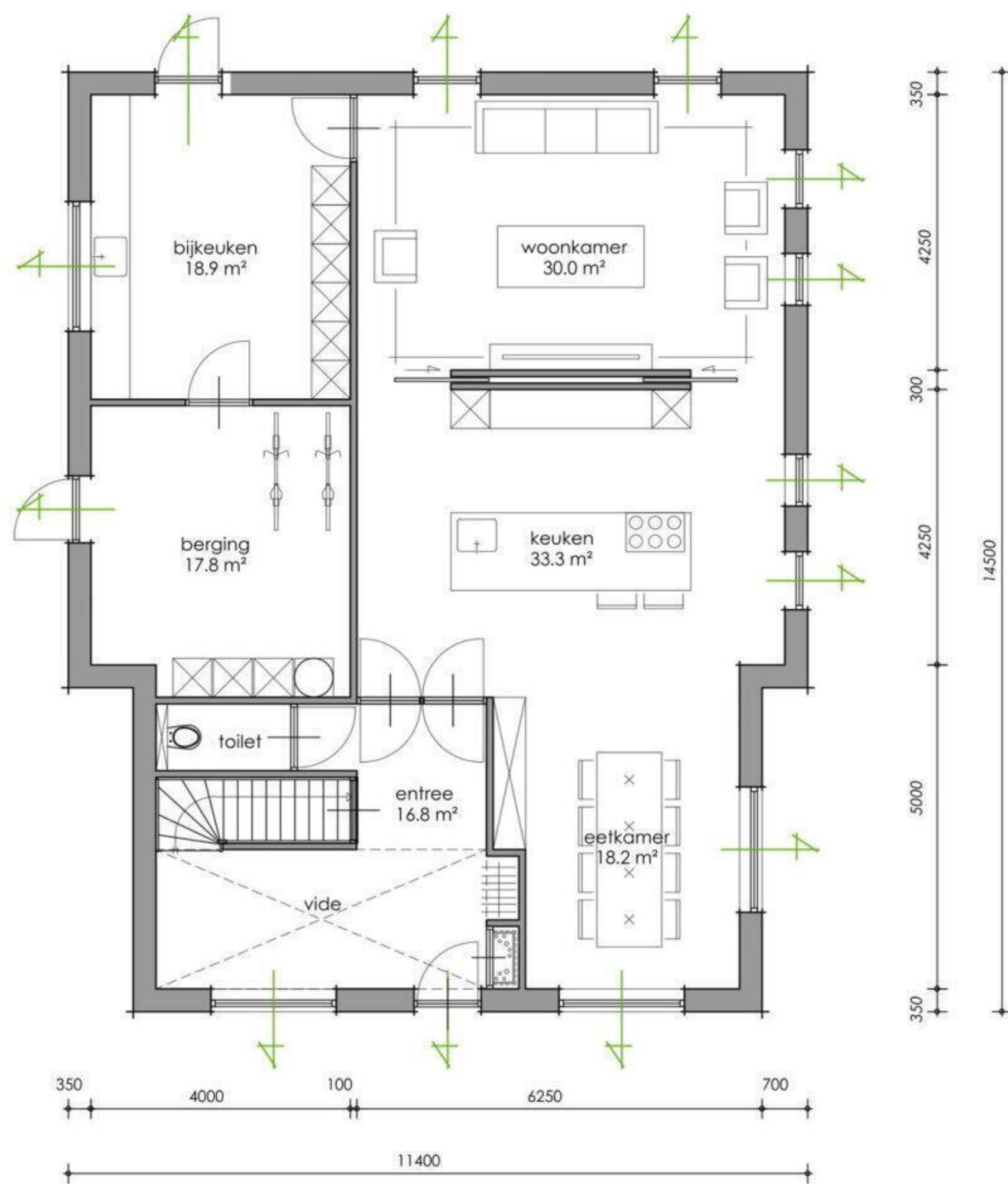
BEGANE GROND
