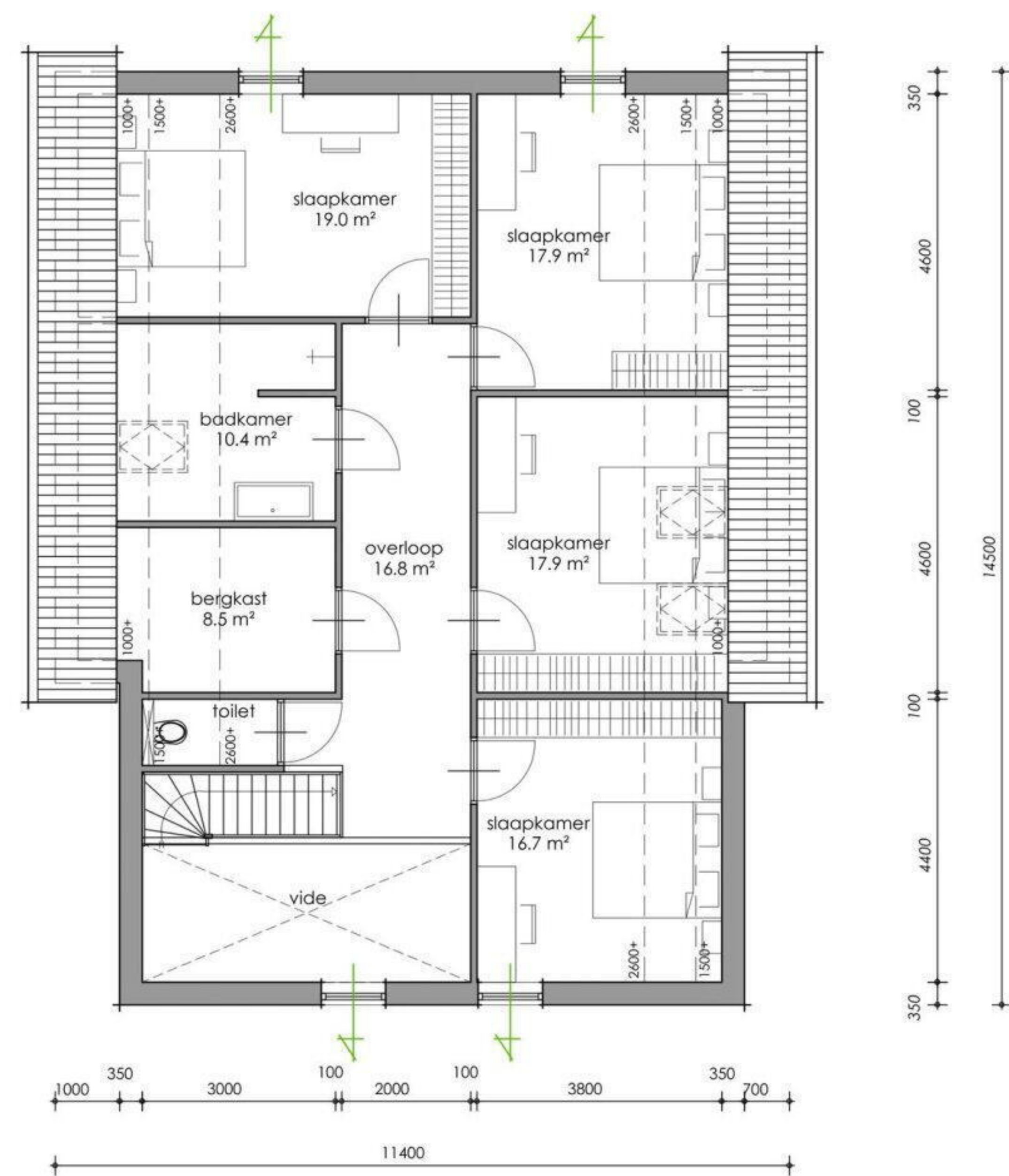
VERDIEPING
