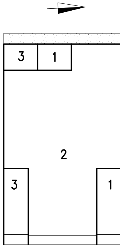
BEGANE GROND schaal 1 : 200
