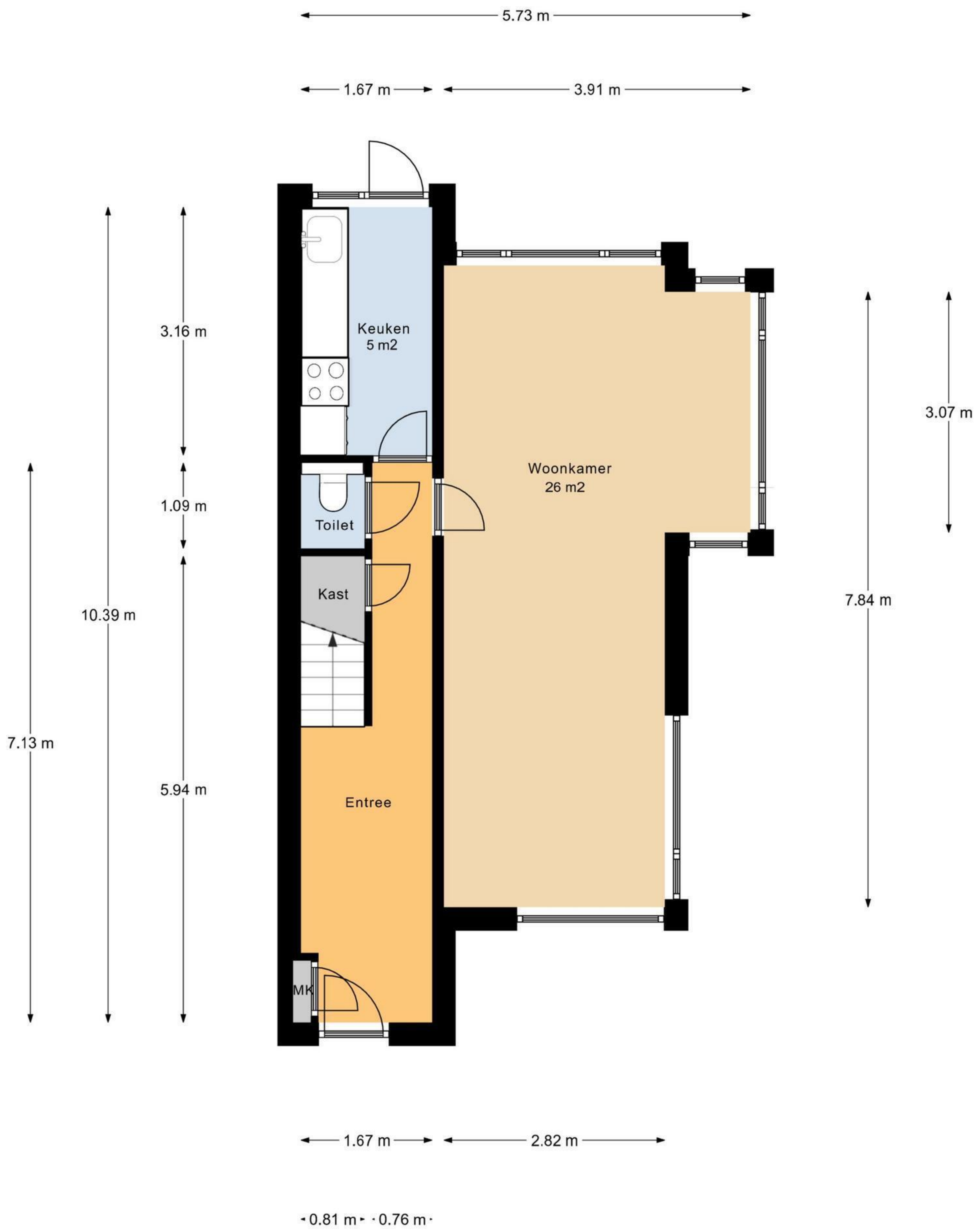
Begane Grond
