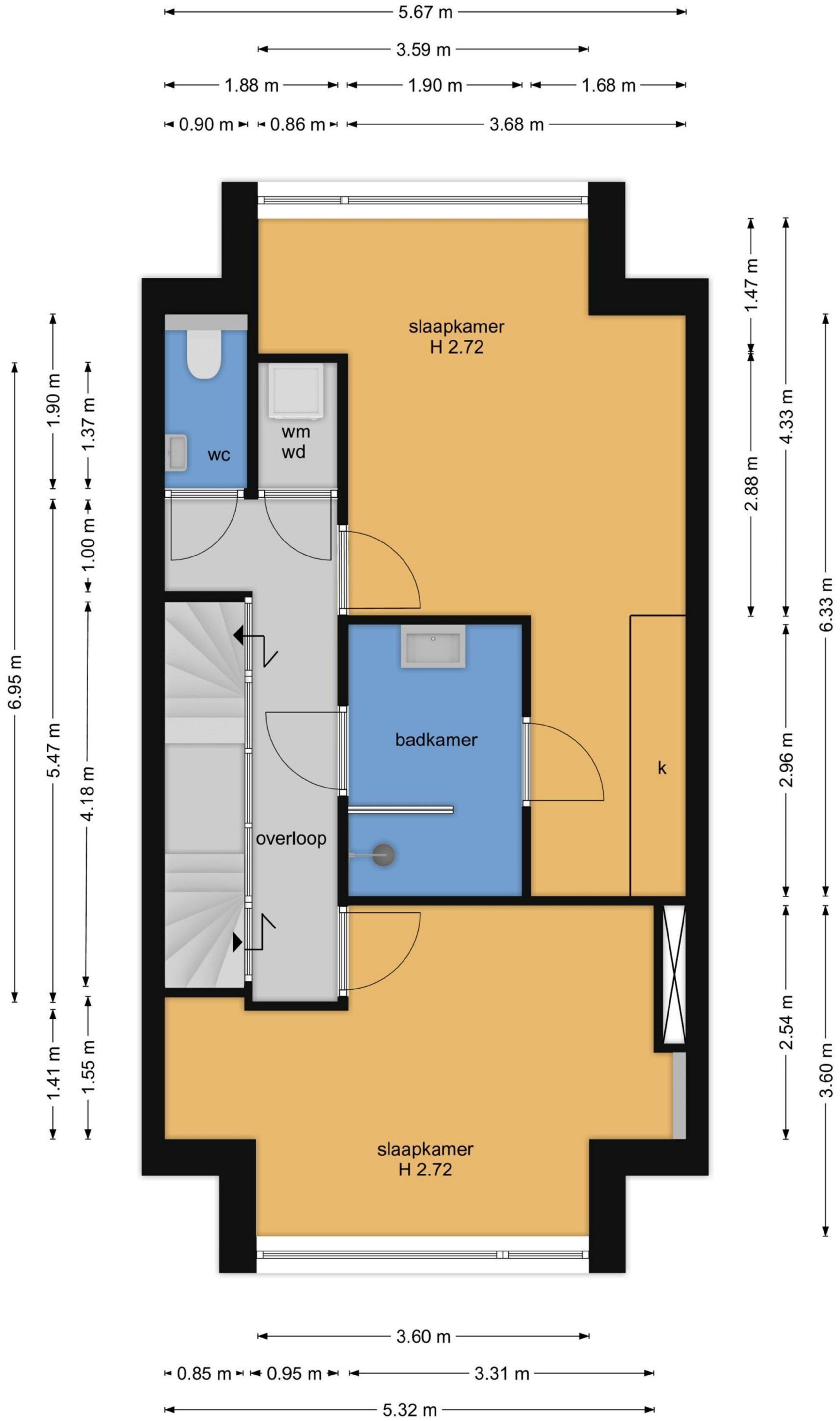
1e verdieping
