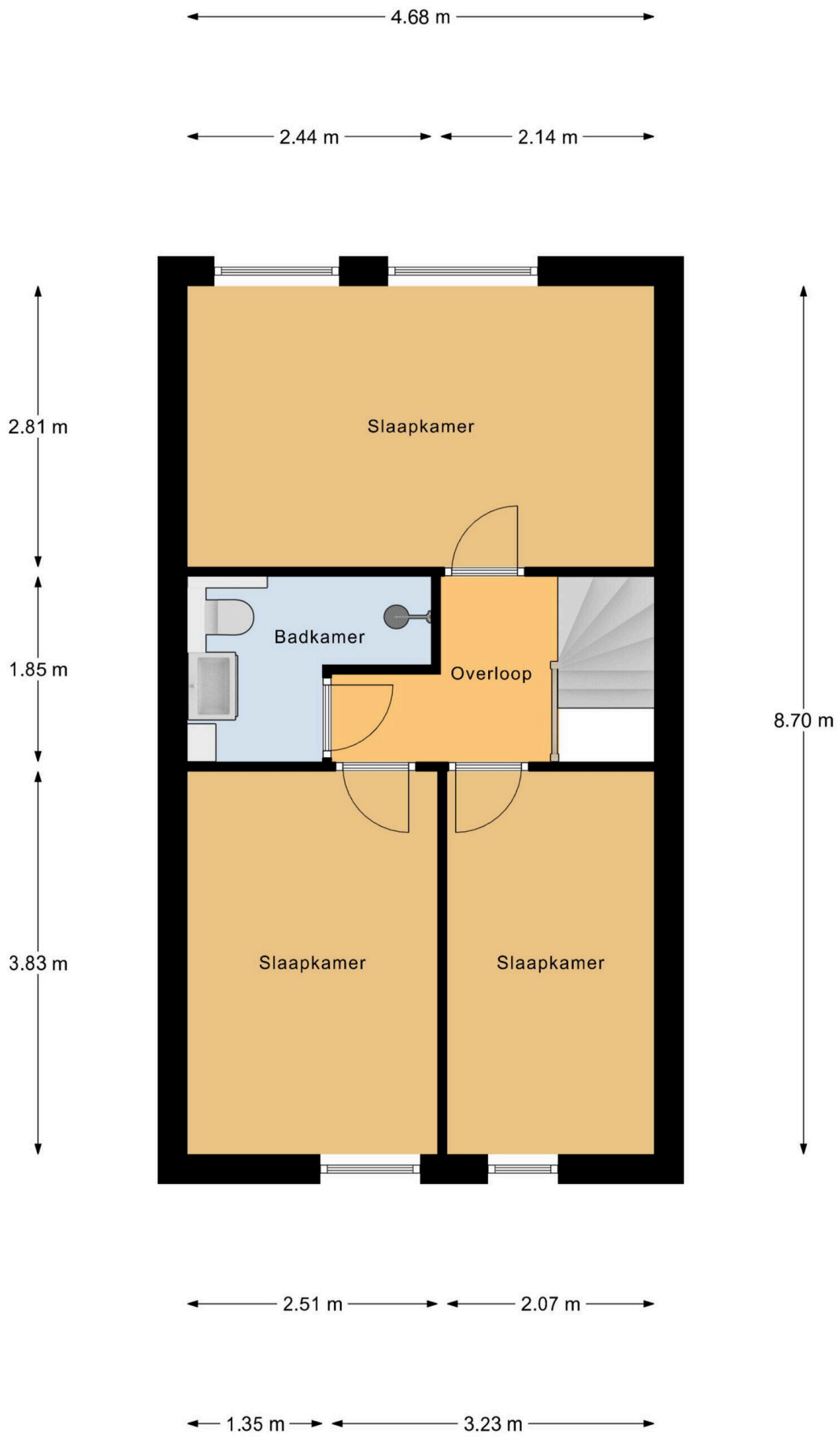
1e Verdieping
