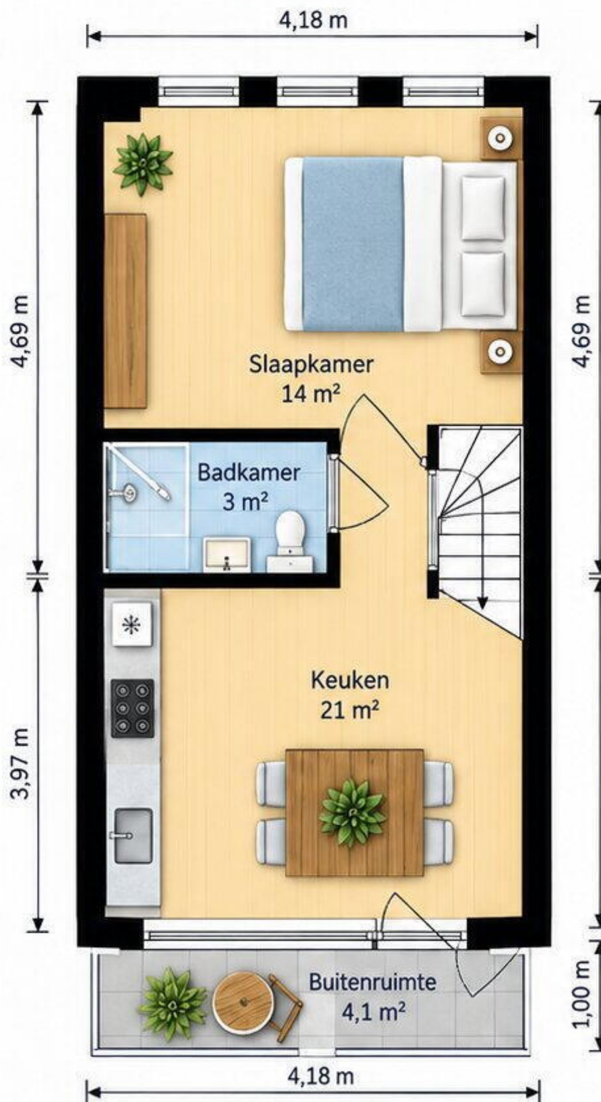
1e verdieping
