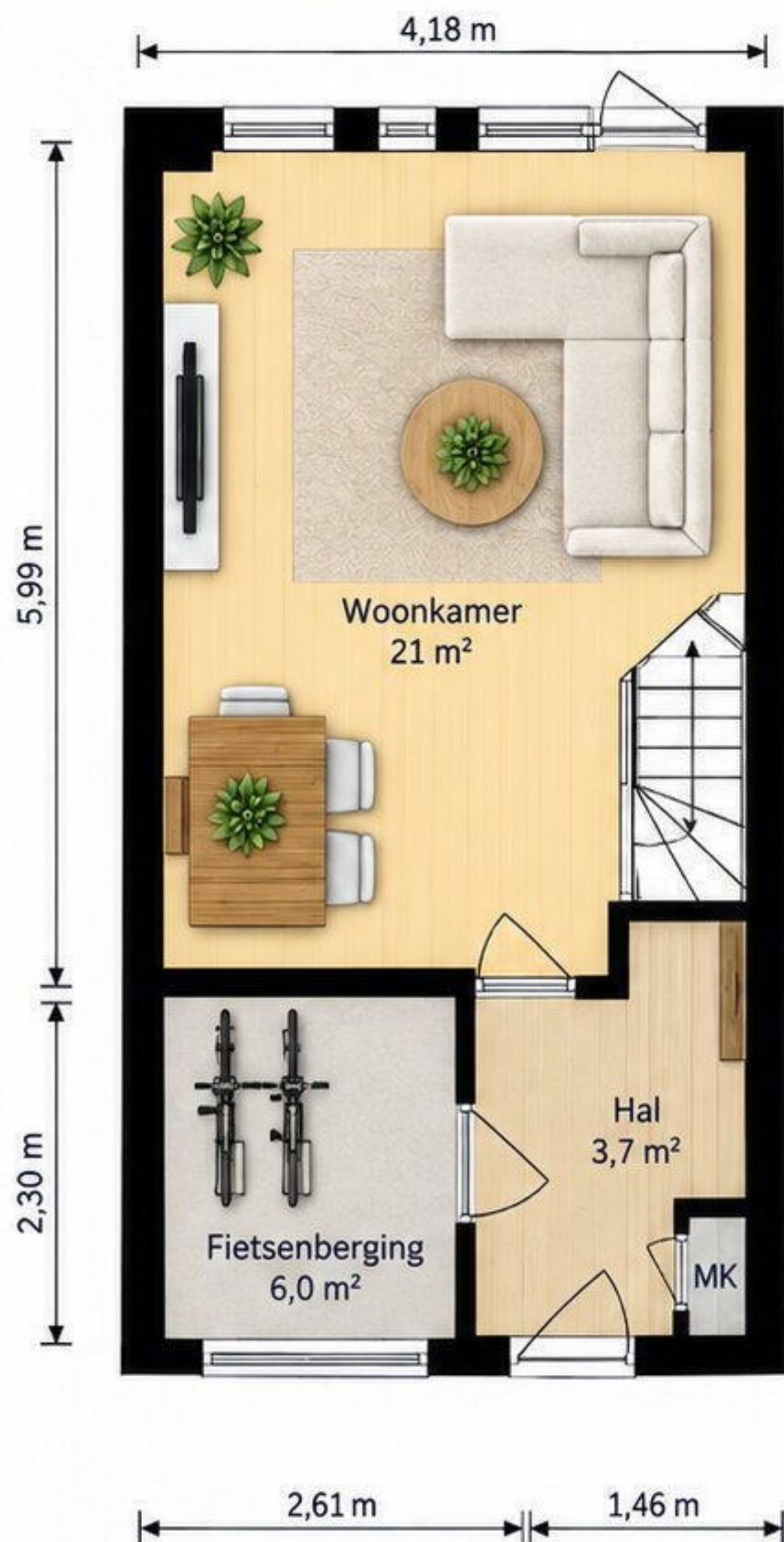
Begane grond
