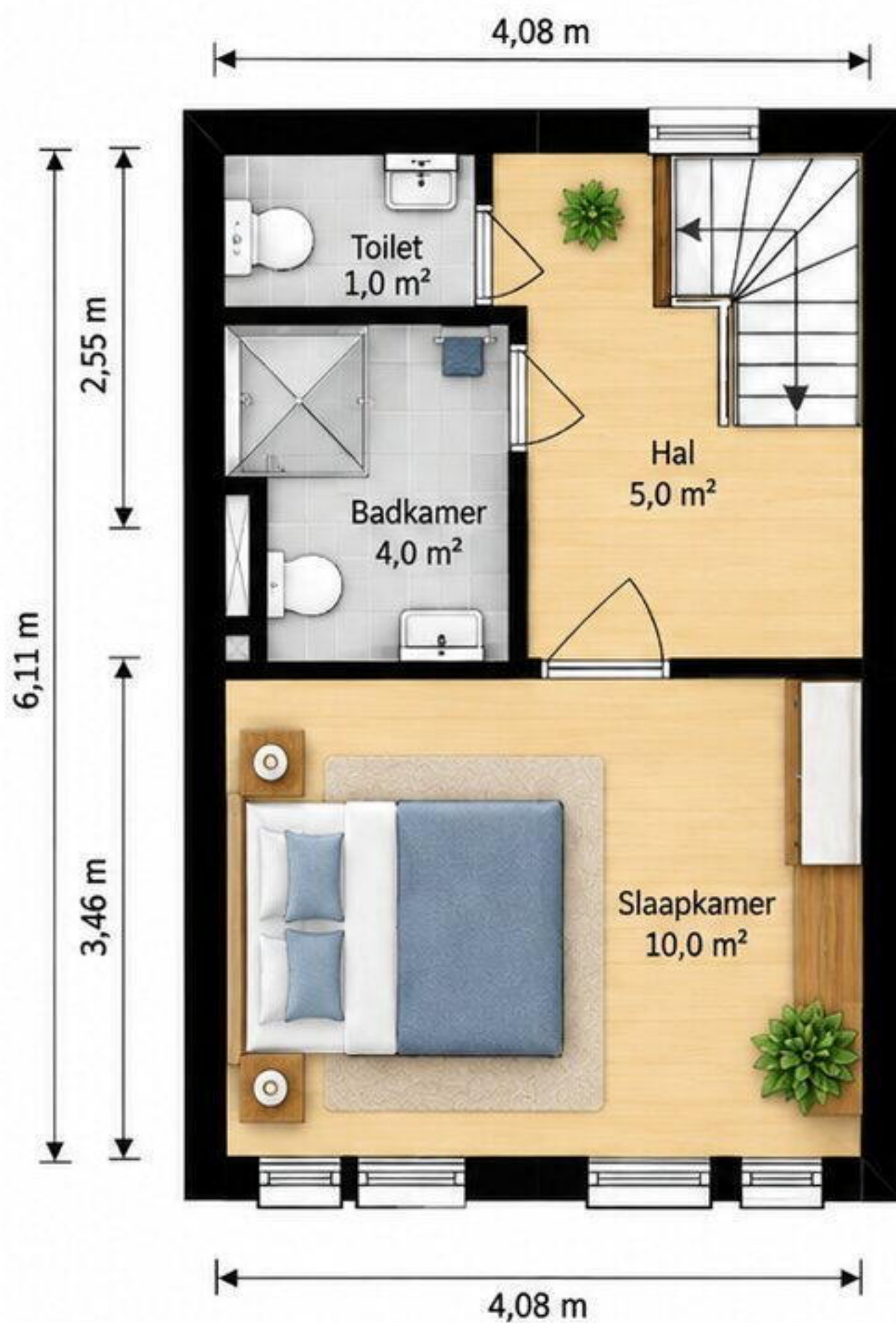
2e verdieping
