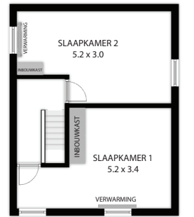
EERSTE VERDIEPING
