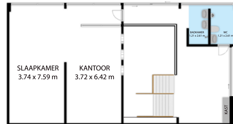
BEGANE GROND
