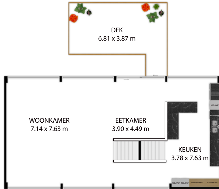
EERSTE VERDIEPING
