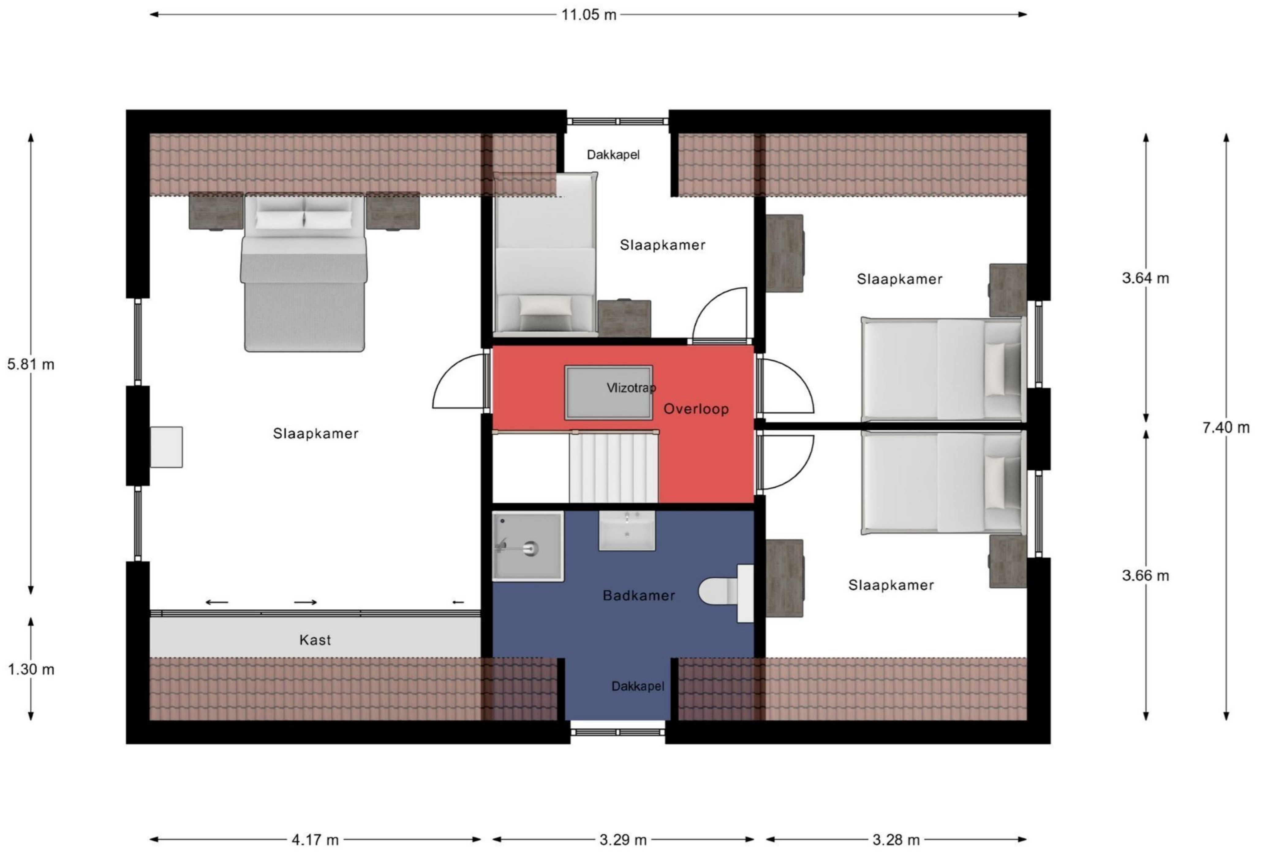
Eerste Verdieping
