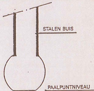
VARIANT GEPULSTE PAAL MET BOLVOET
