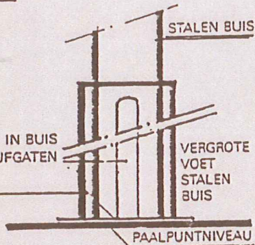
VARIANT GEHEIDE PAAL MET VERZWAARDE VOET
