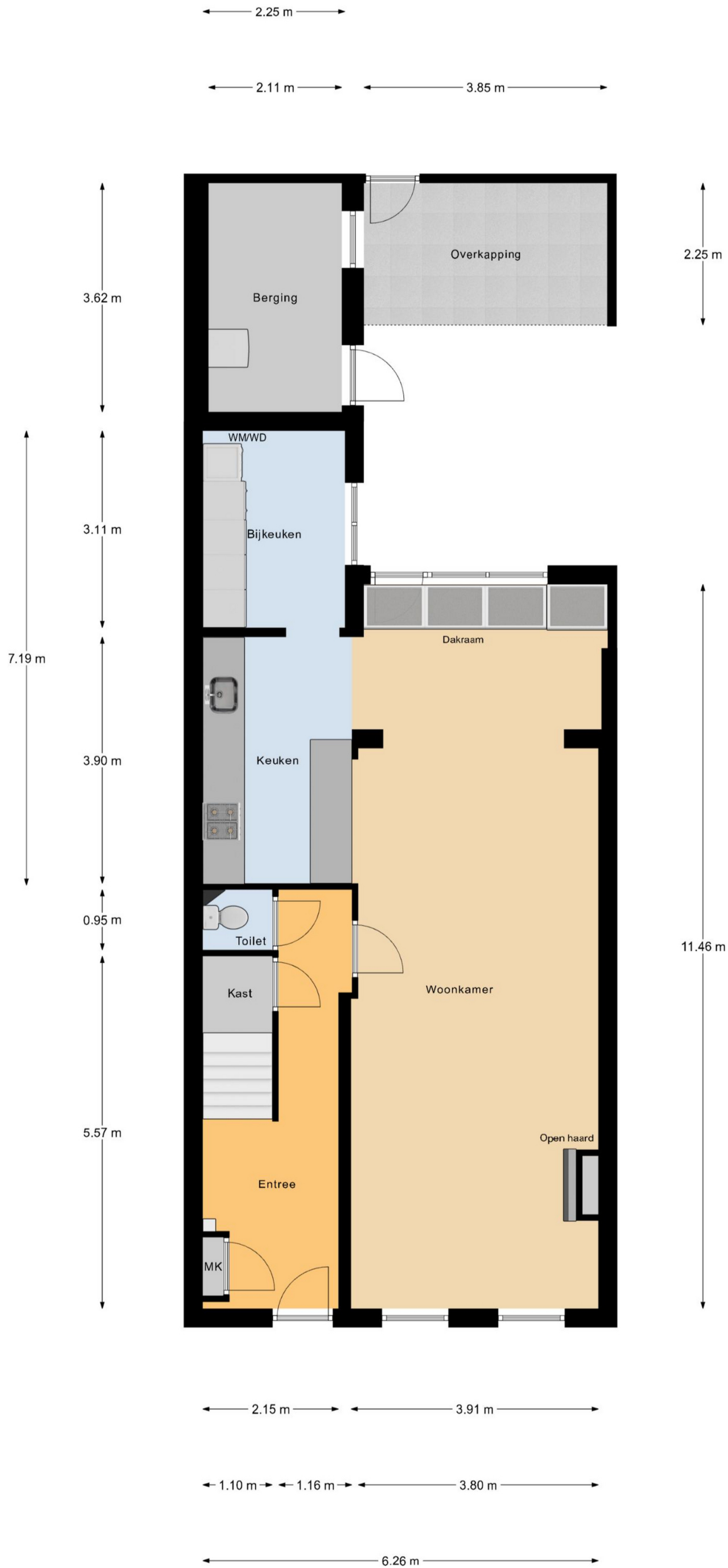
Begane Grond
