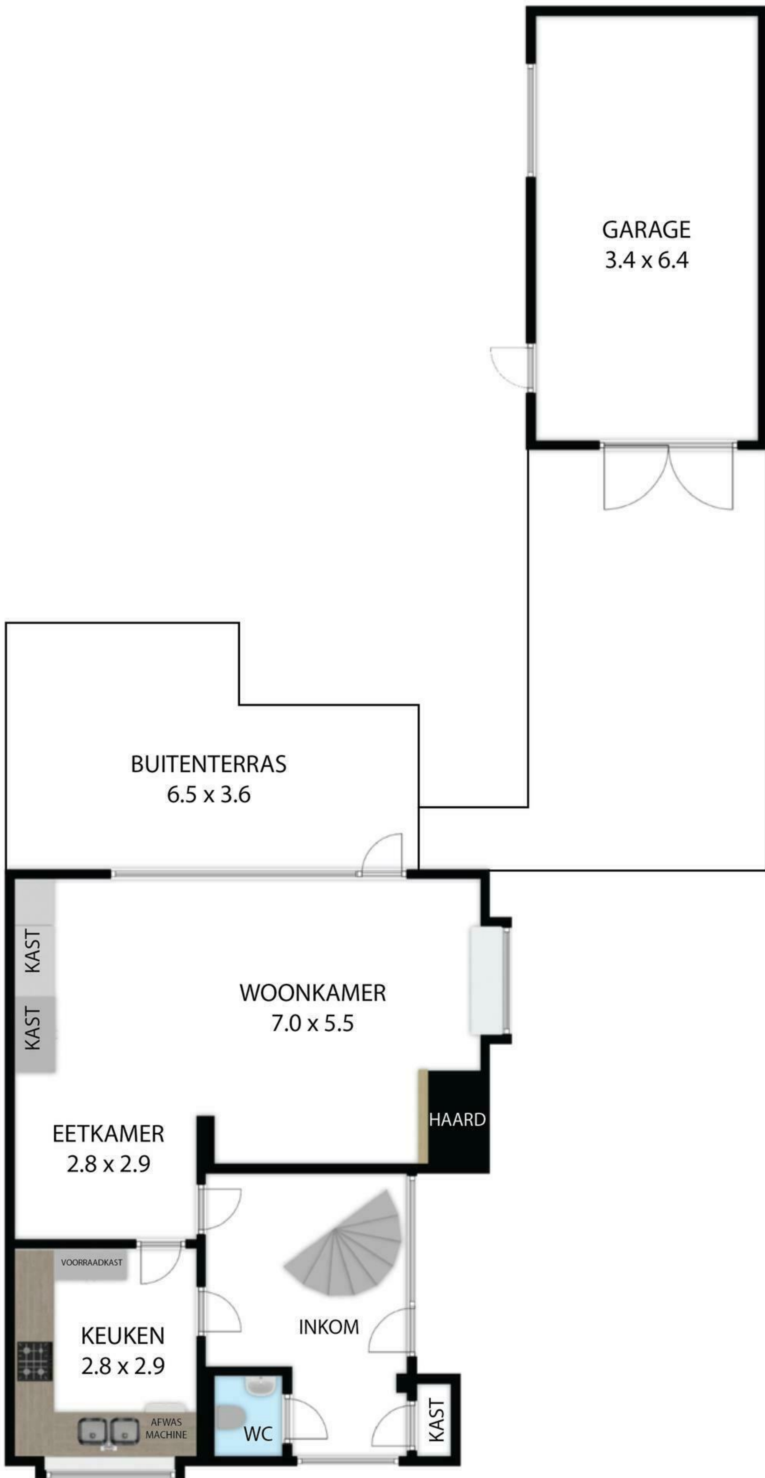
BEGANE GROND
