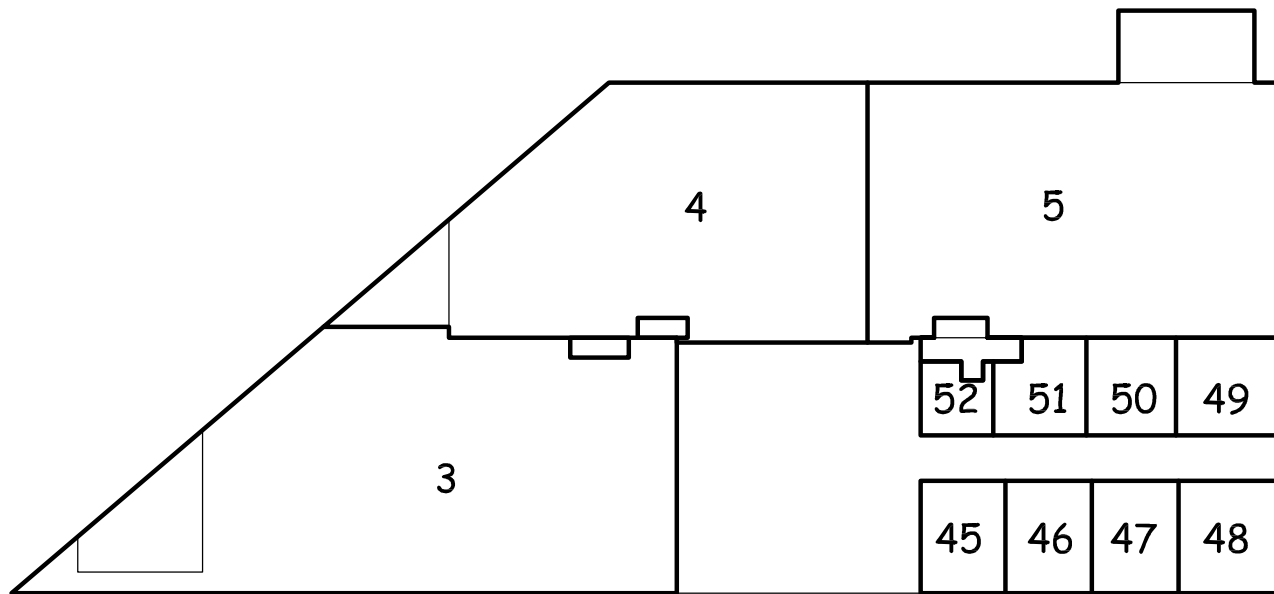
1E VERDIEPING - schaal 1:200
