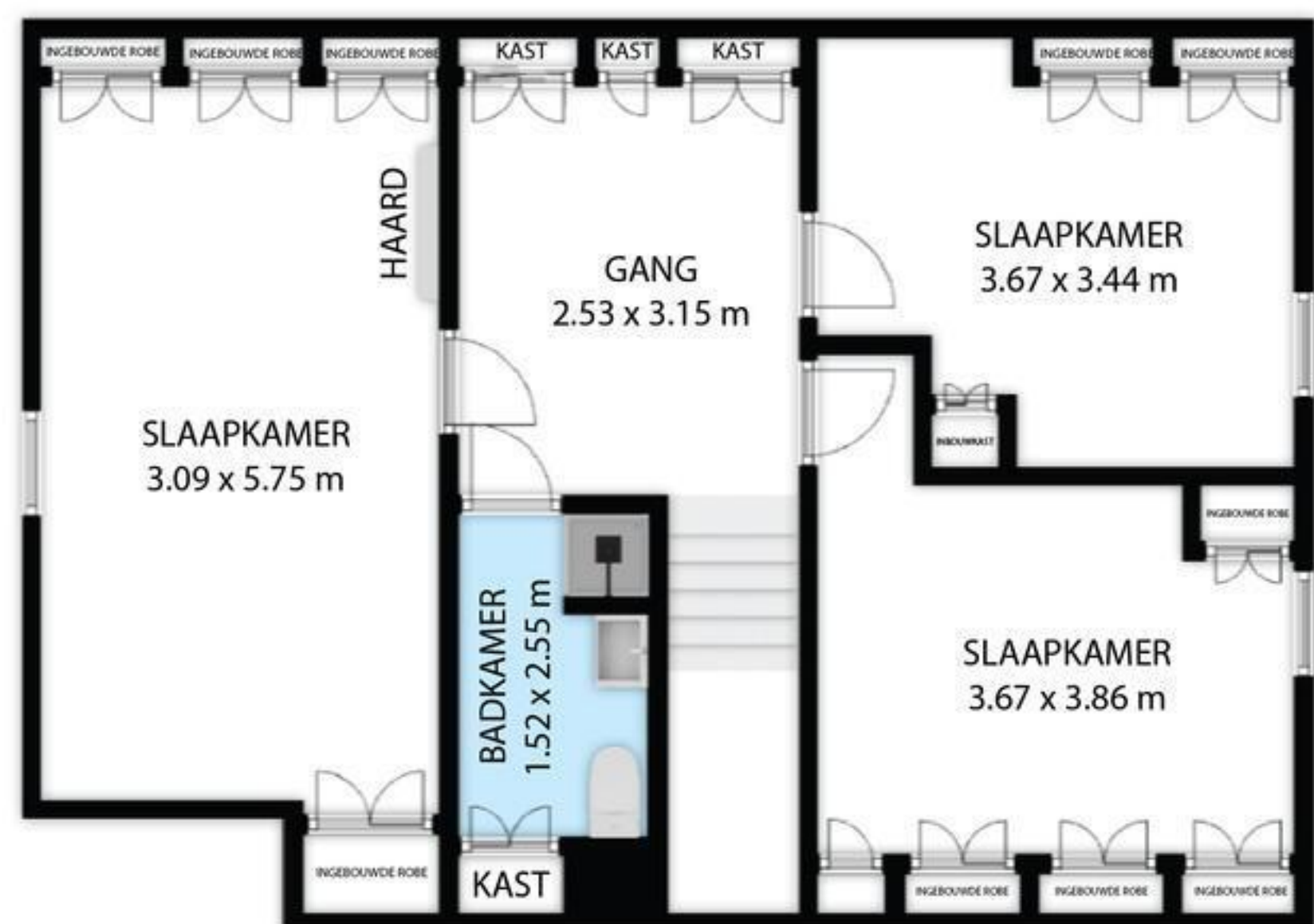
EERSTE VERDIEPING
