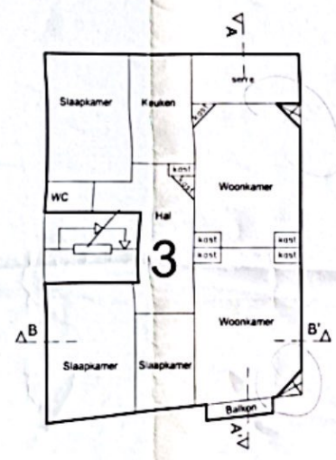
2e Verdieping 1:100
