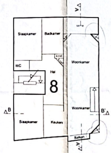
3e Verdieping 1:100
