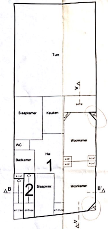
Begane Grond 1:100
