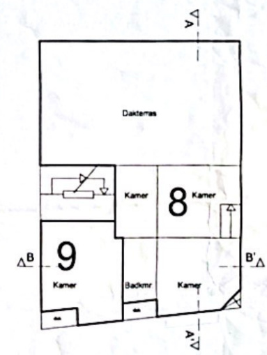
4e Verdieping 1:100
