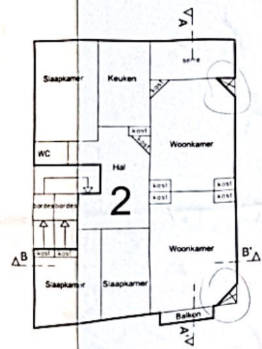
1e Verdieping 1:100
