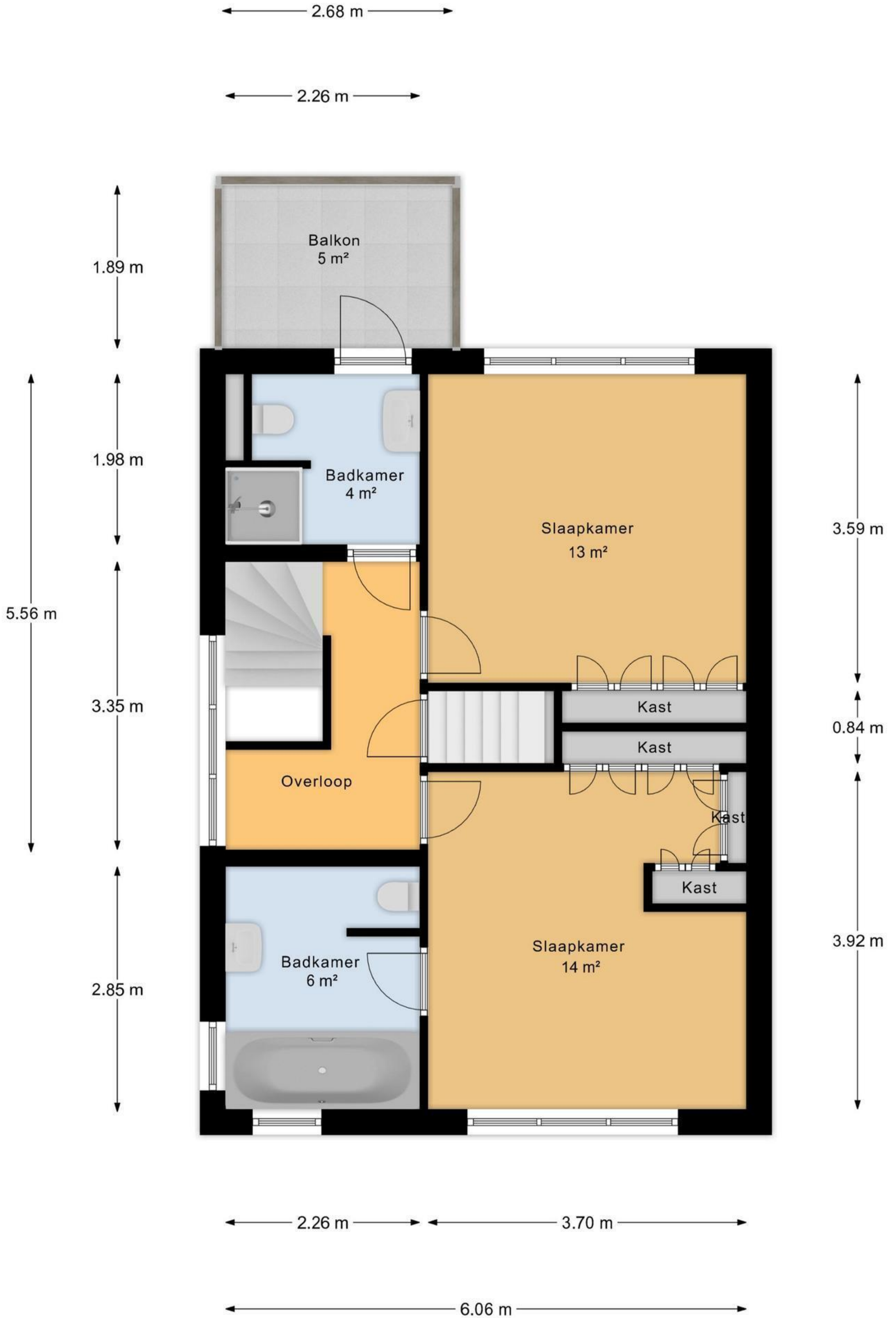
Eerste Verdieping
