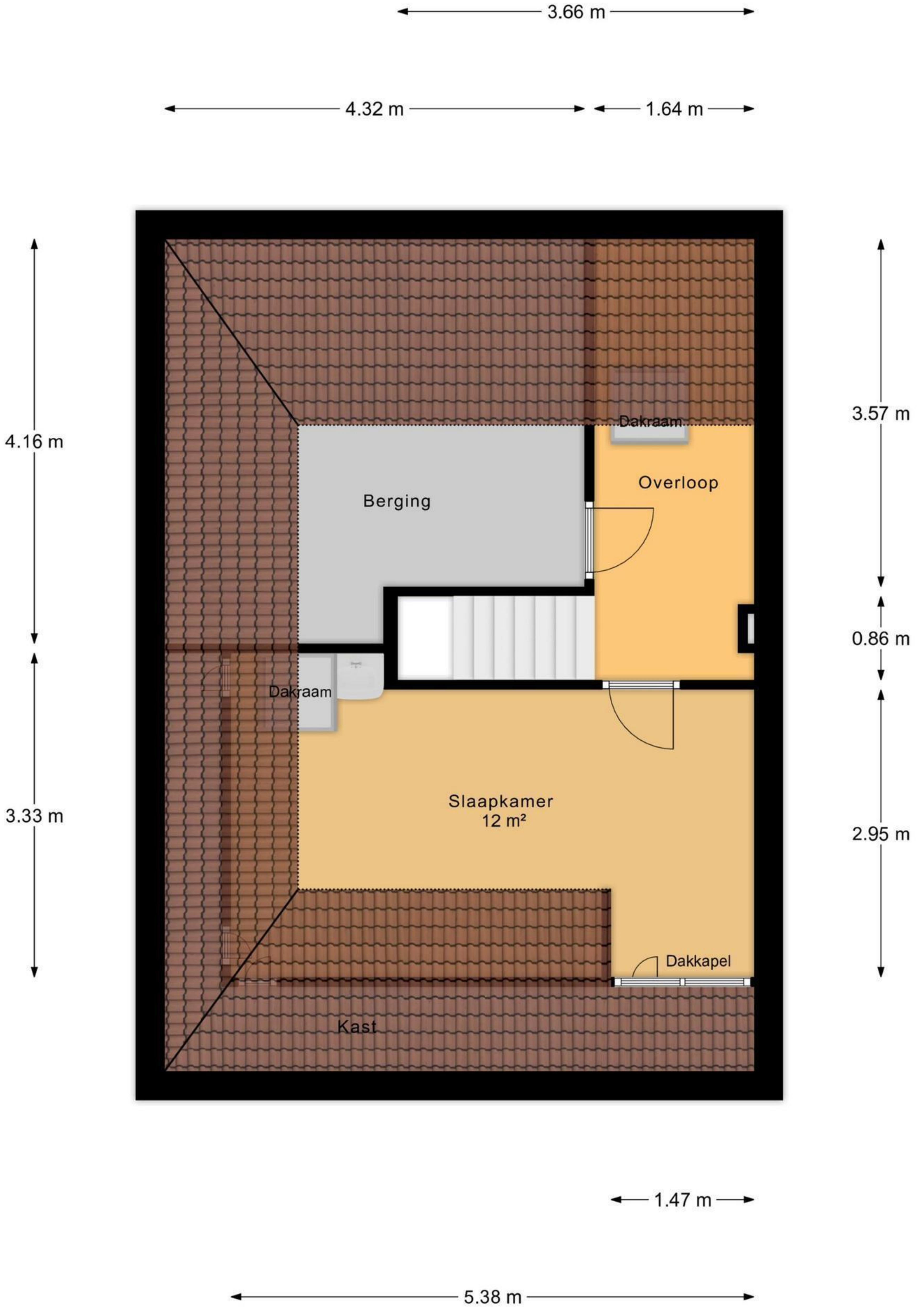
Tweede Verdieping
