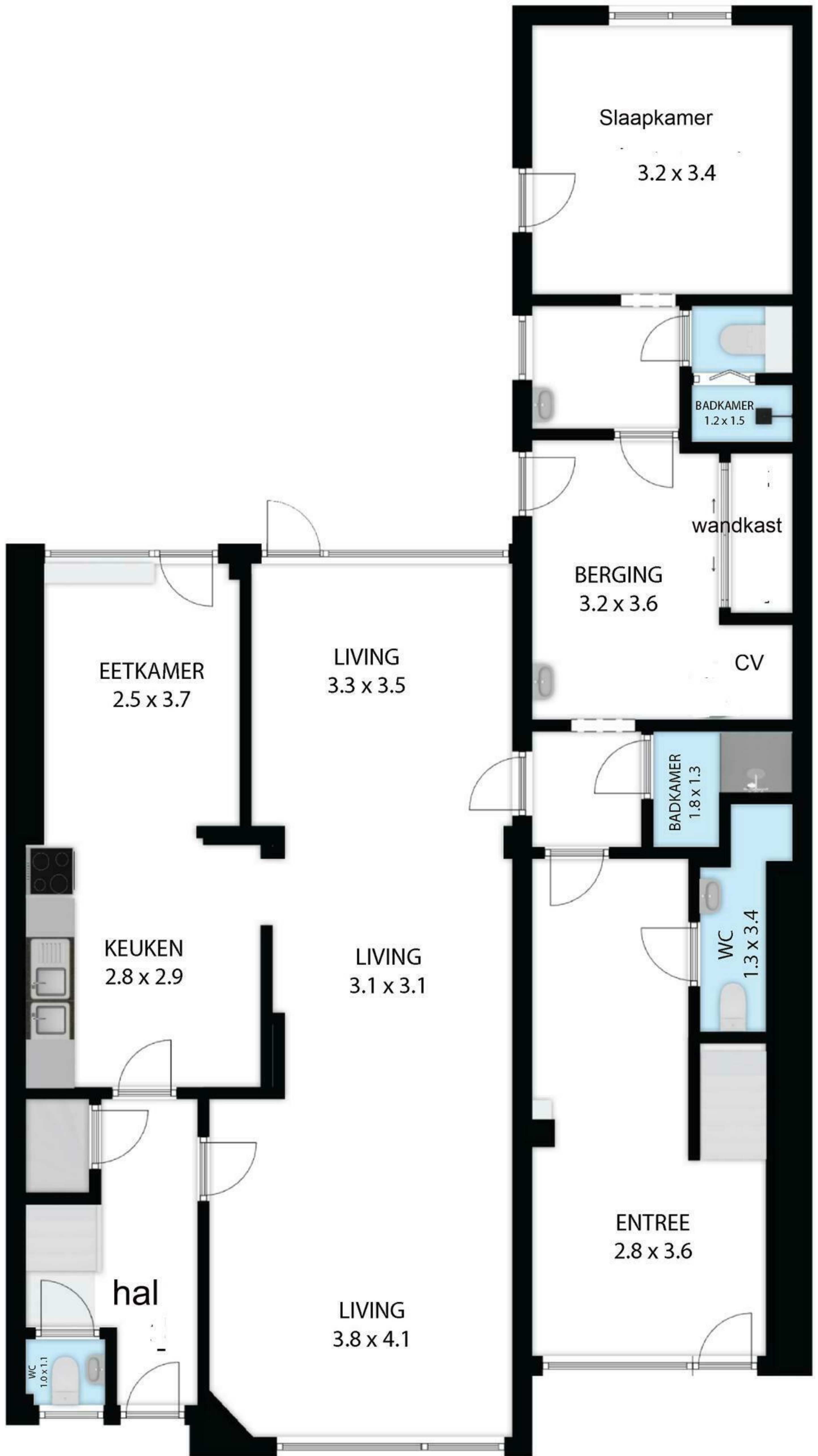
BEGANE GROND
