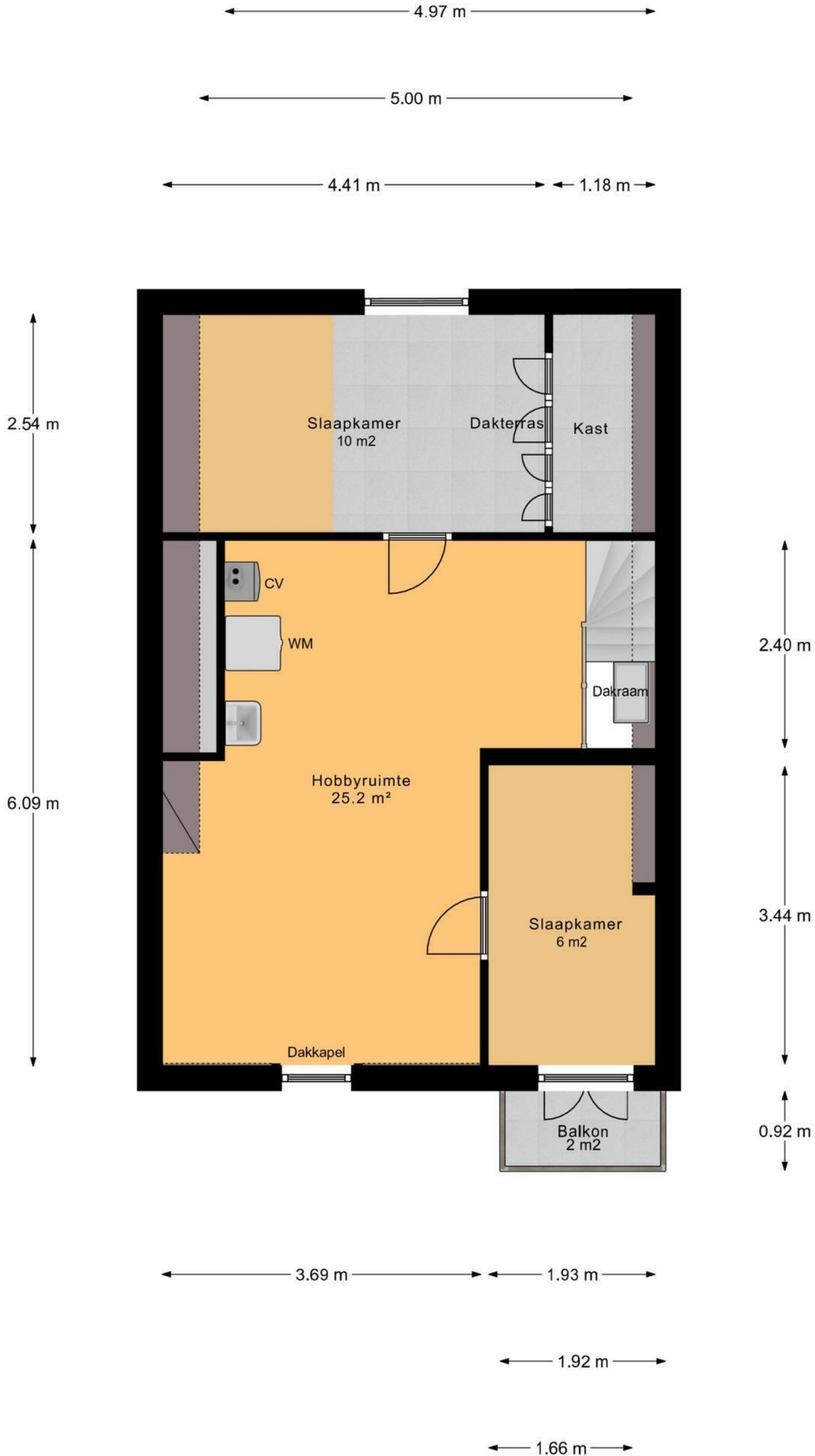
2e Verdieping
