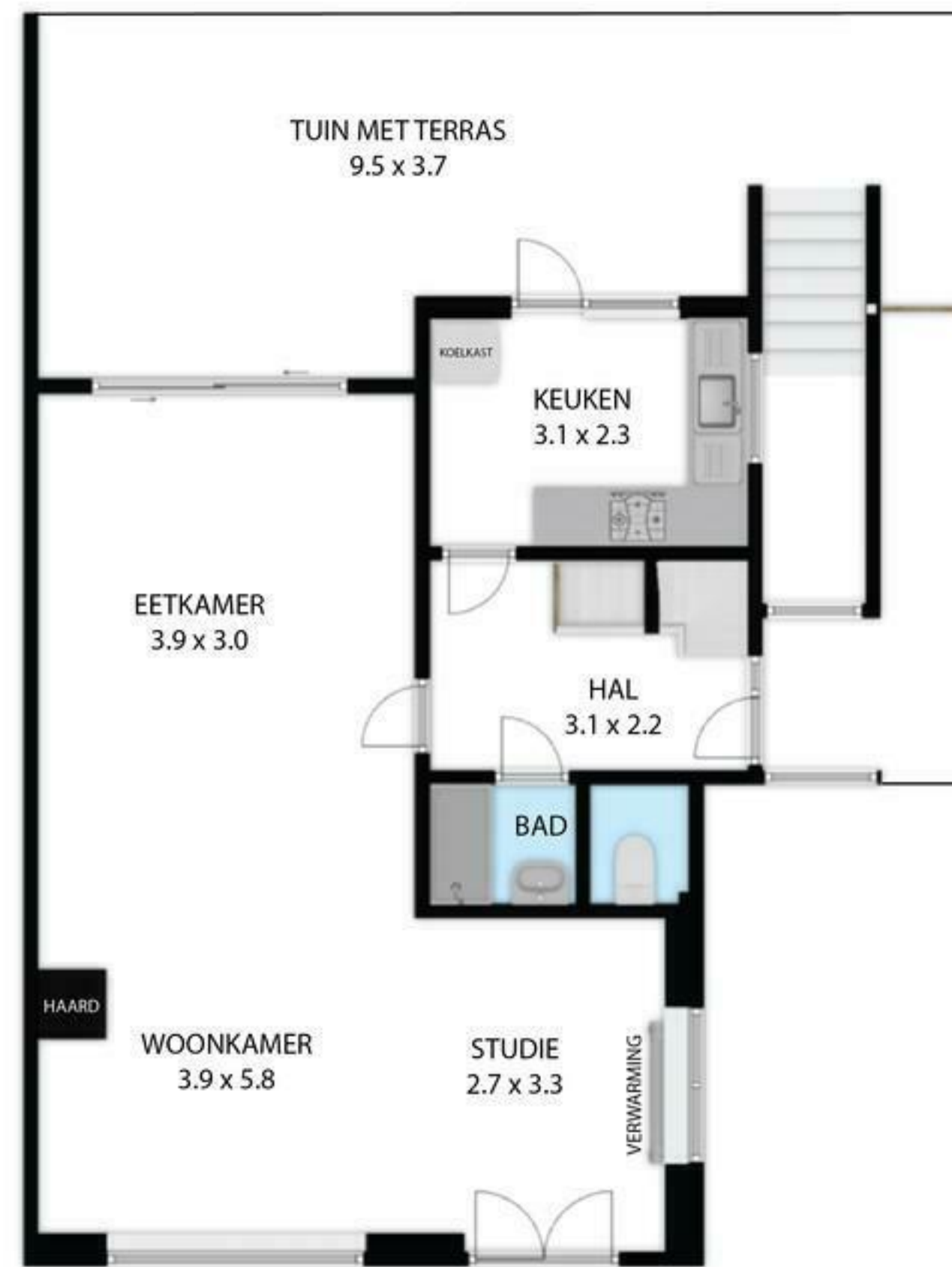
BEGANE GROND
