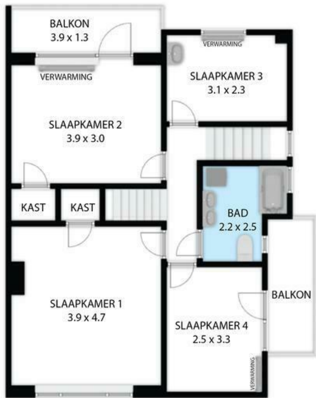
EERSTE VERDIEPING
