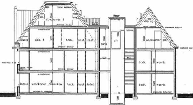
-doorsnede B-B-
