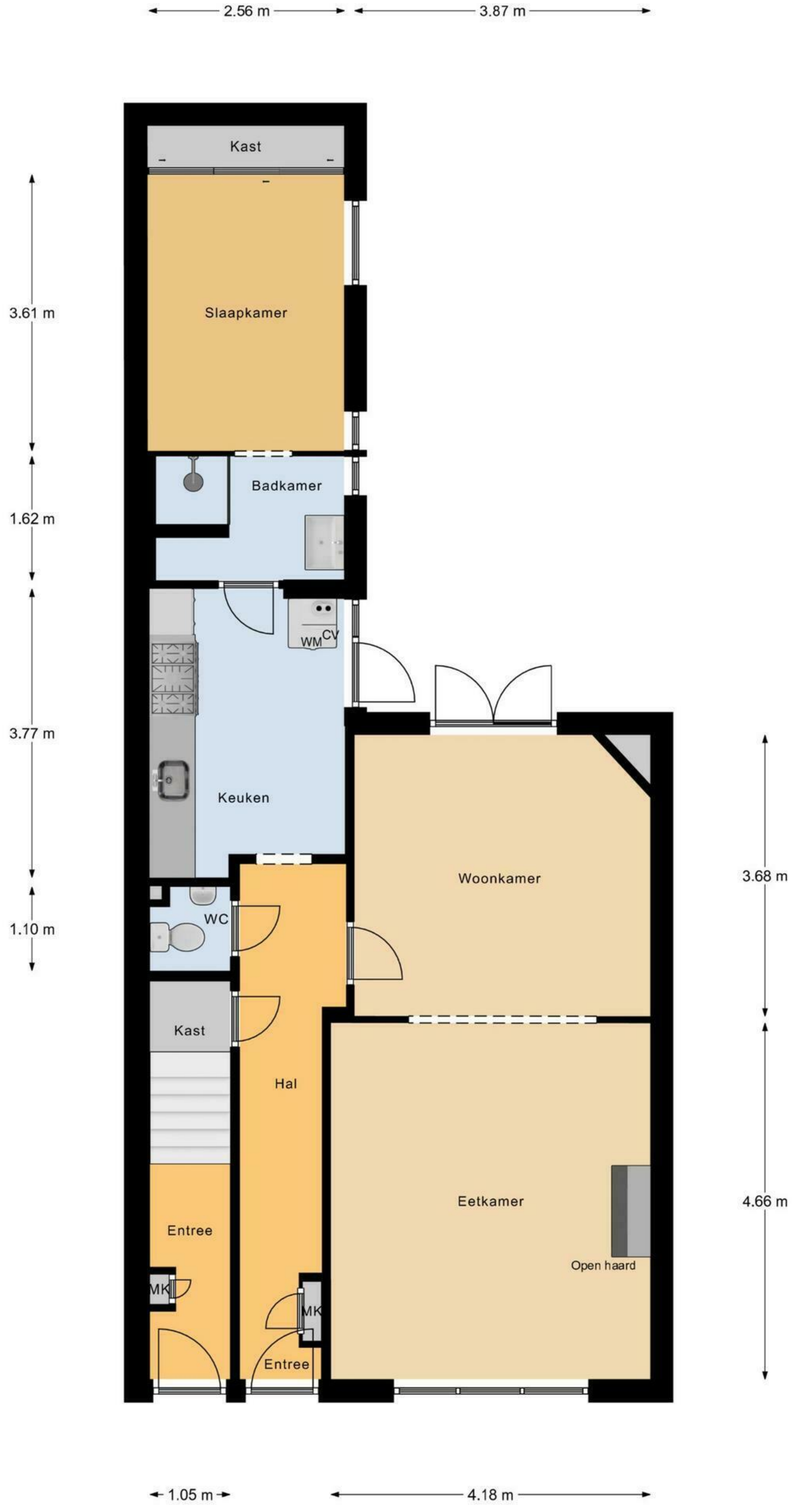
Begane Grond
