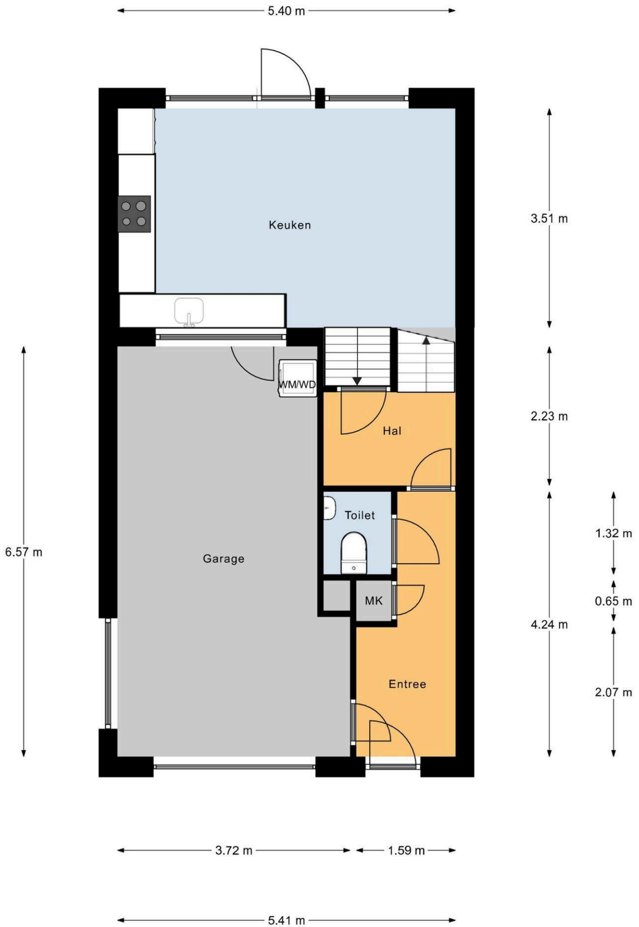
Begane Grond
