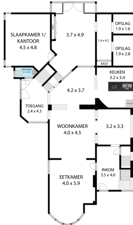
BEGANE GROND
