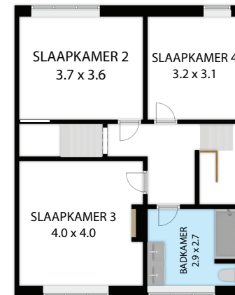
EERSTE VERDIEPING
