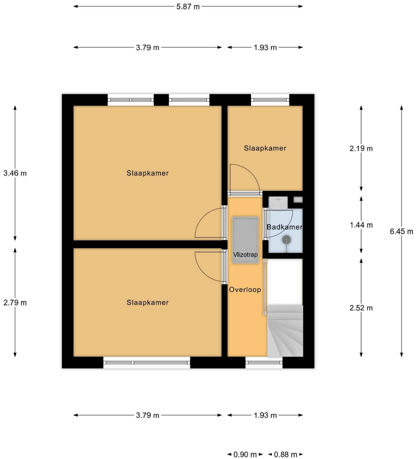
1e Verdieping
