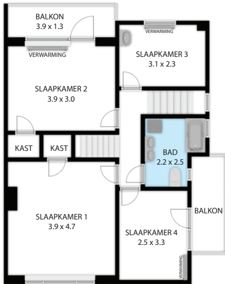
EERSTE VERDIEPING
